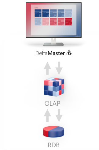
OLAP
